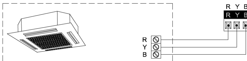
Figura 2. Conexión del KLIC-LG1 a la máquina de A/A.
