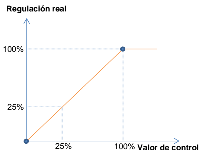
Figura 11. Curva de control por defecto.
