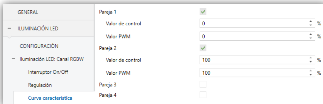
Figura 14. Curva Característica
