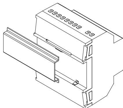
Figura 3: Montaje de HeatingBOX 24V 8X en carril DIN
