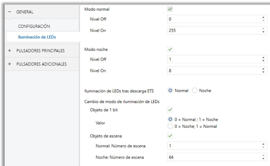
Figura 30. General - Iluminación de LEDs: Modo noche.
