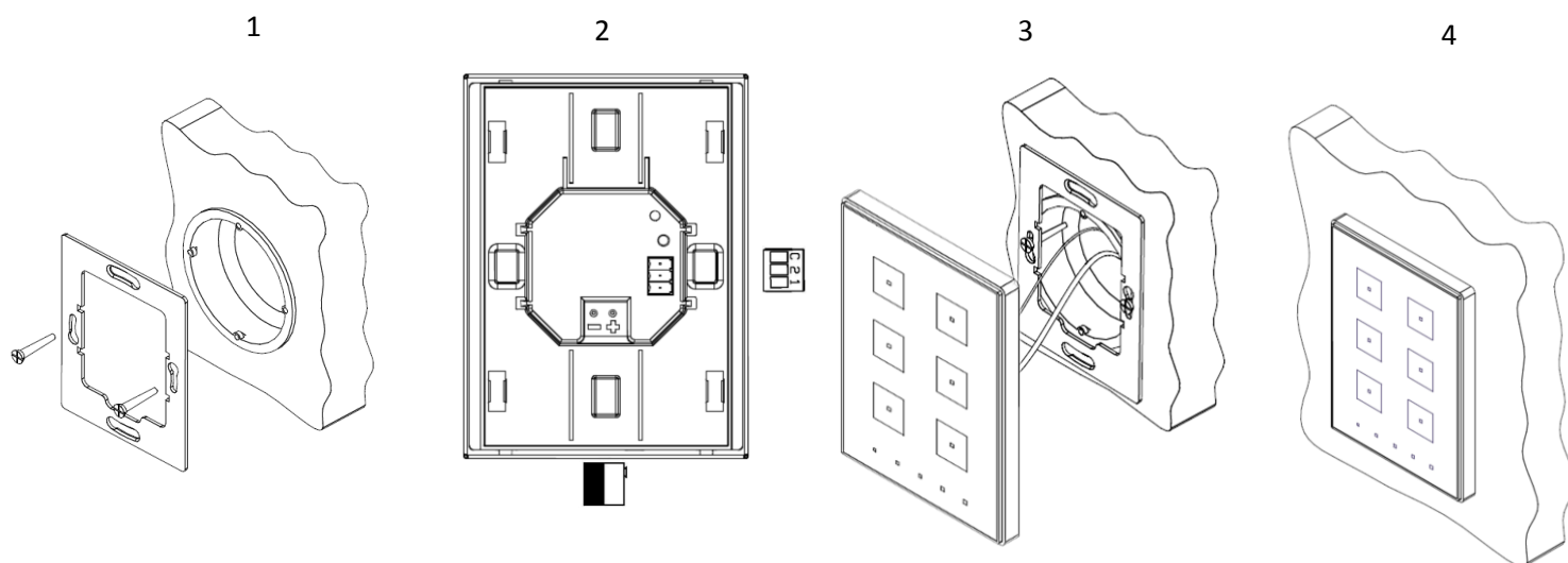
Figura 2. Instalación del Touch-MyDesign Plus.
