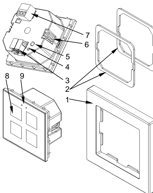
Figura 2 Diagrama de elementos de Flat 55.
