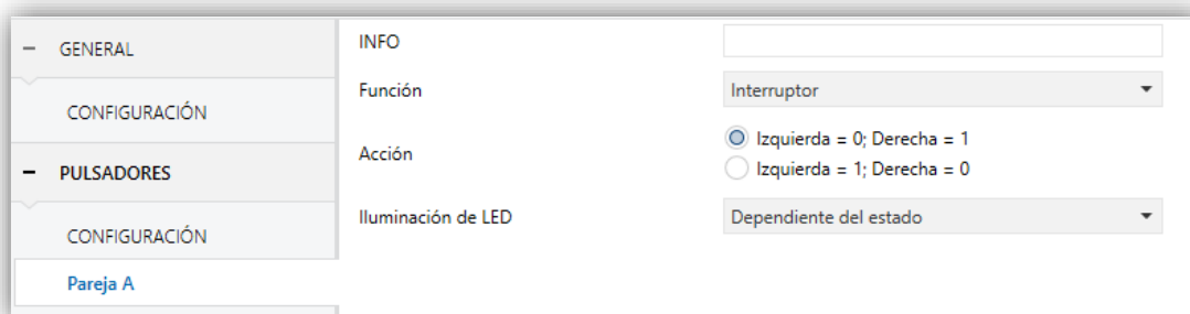
Figura 29 Pareja de pulsadores - Interruptor.
