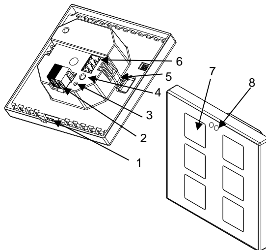
Figura 1 Diagrama de elementos de Flat.
